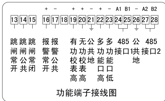
外置负荷开关电能表功能端子接线图
