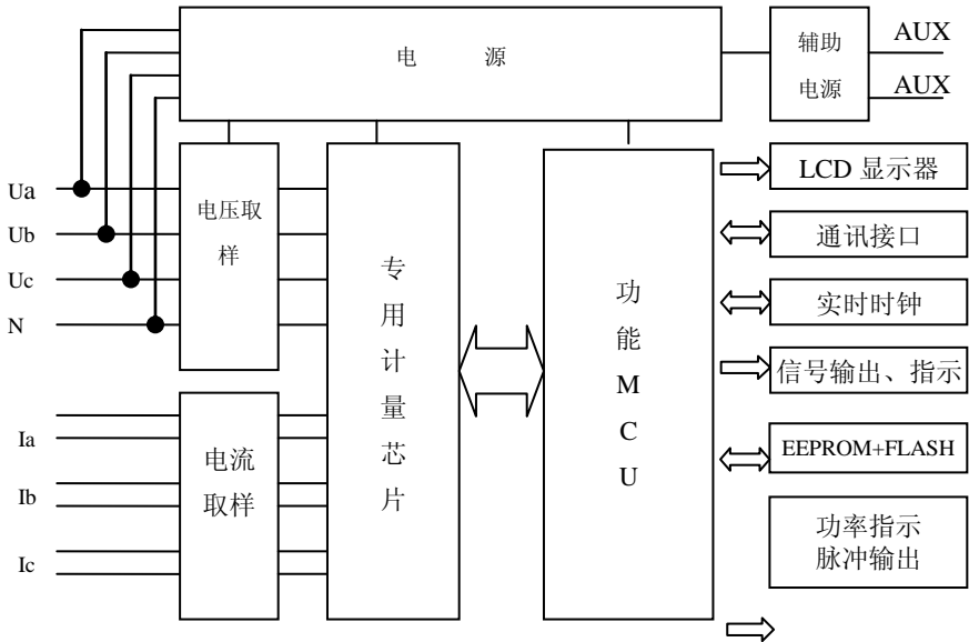
原理框图
